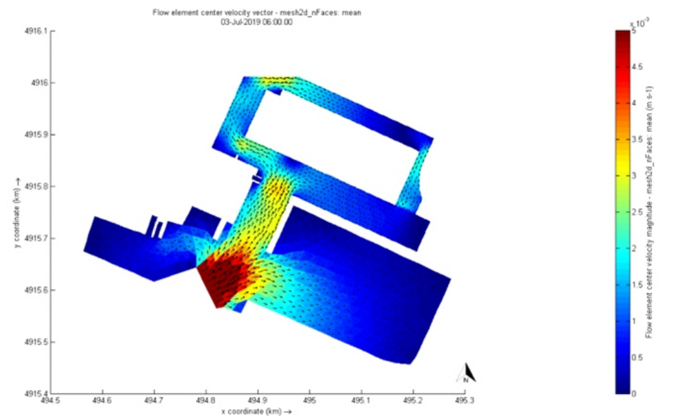
Modello idrodinamico a supporto del progetto di recupero del waterfront, Genova - Comune di Genova
